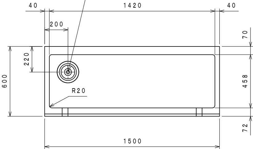
大型ゴミ収納器付防臭排水トラップ（４０Ａ）
