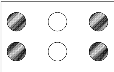
φ180二重バーナ インพุット配置図
