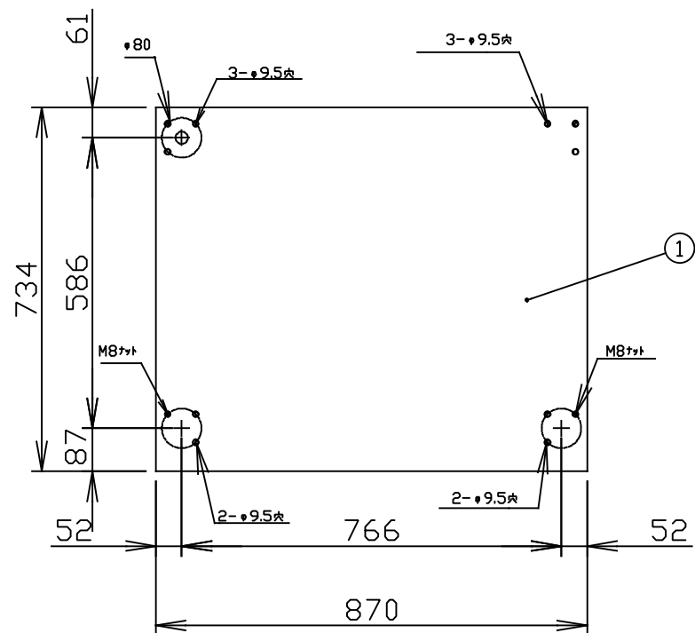
架台C仕様（キャビネット仕様）
