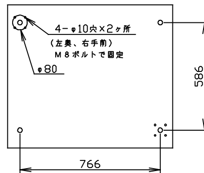
本体耐震調節脚固定穴位置
