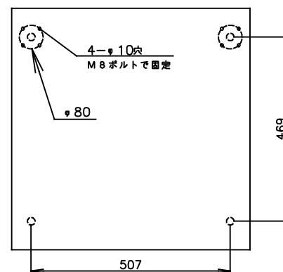
本体耐震調節脚固定穴位置
