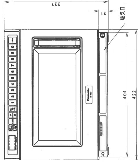
正面図
