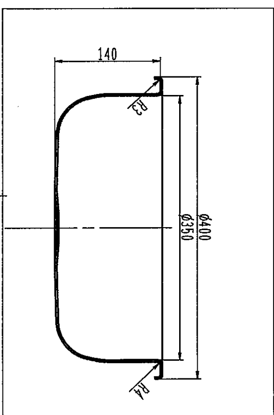
内鍋
