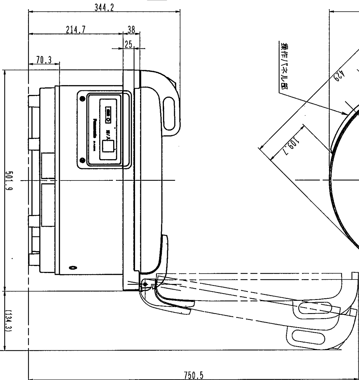
正面図
