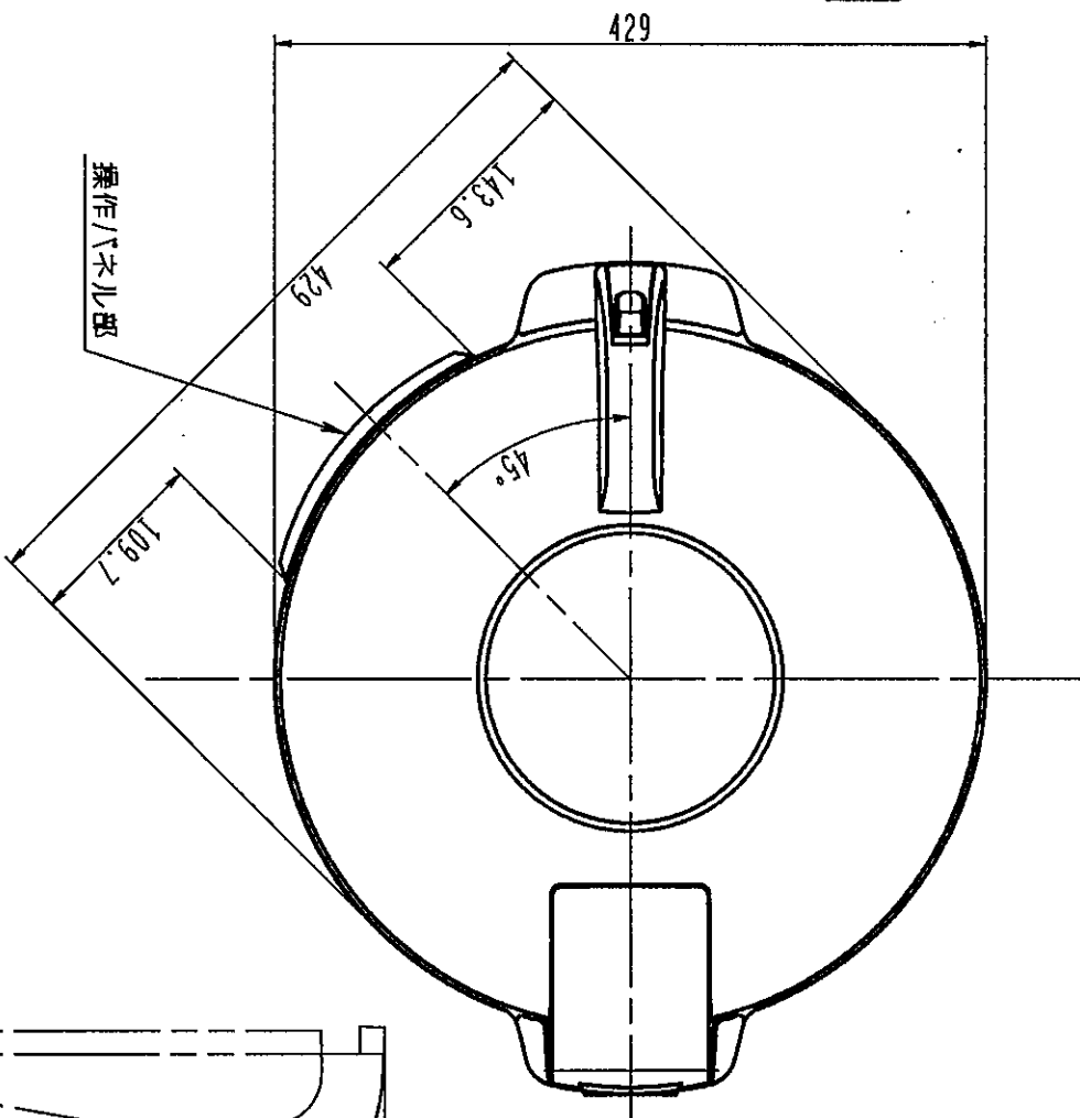
平面図
